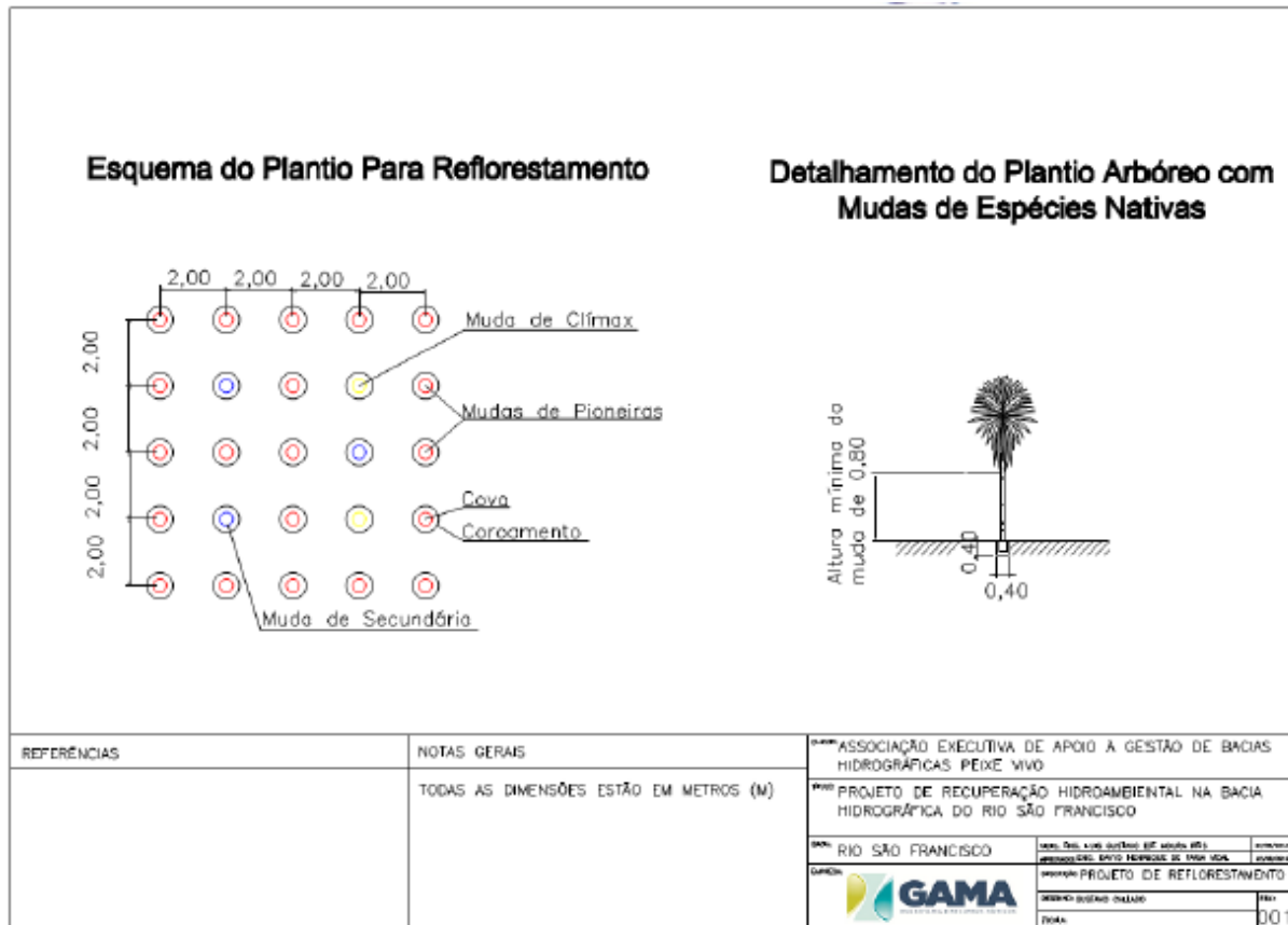
Figura 11: Especificações técnicas para execução do plantio das mudas na área da subbacia do Córrego Siqueiras
