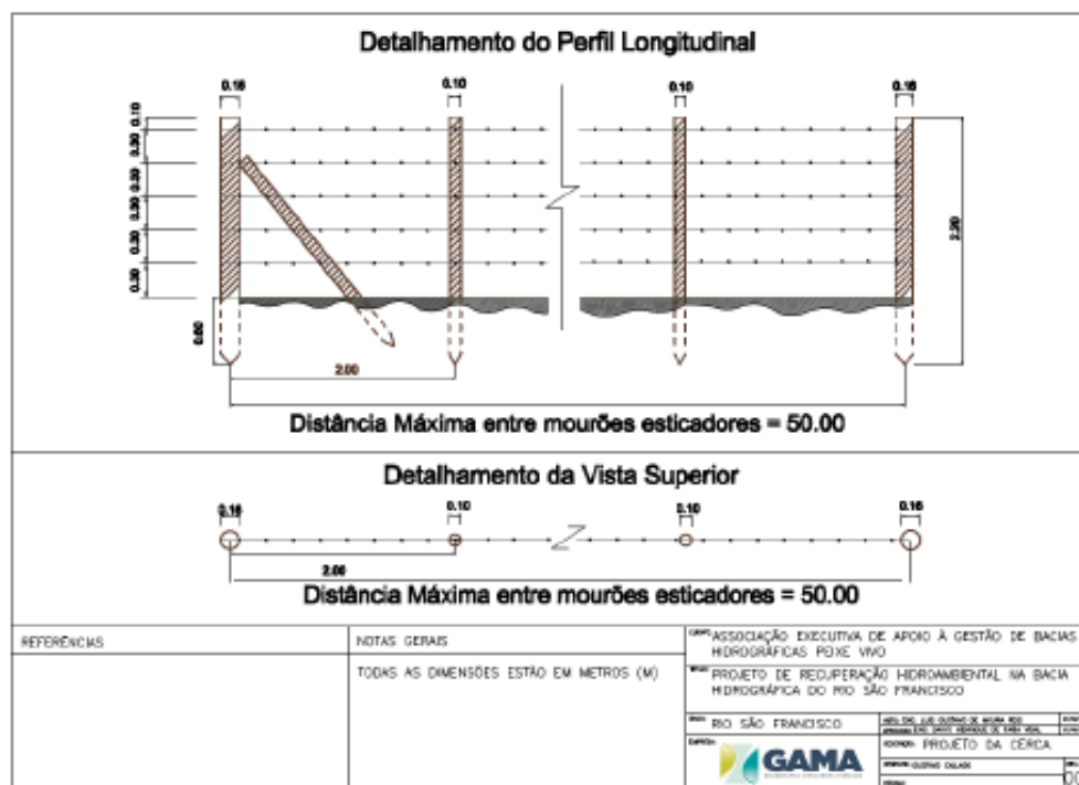
Figura 14: Esquema para cercamento de nascente
